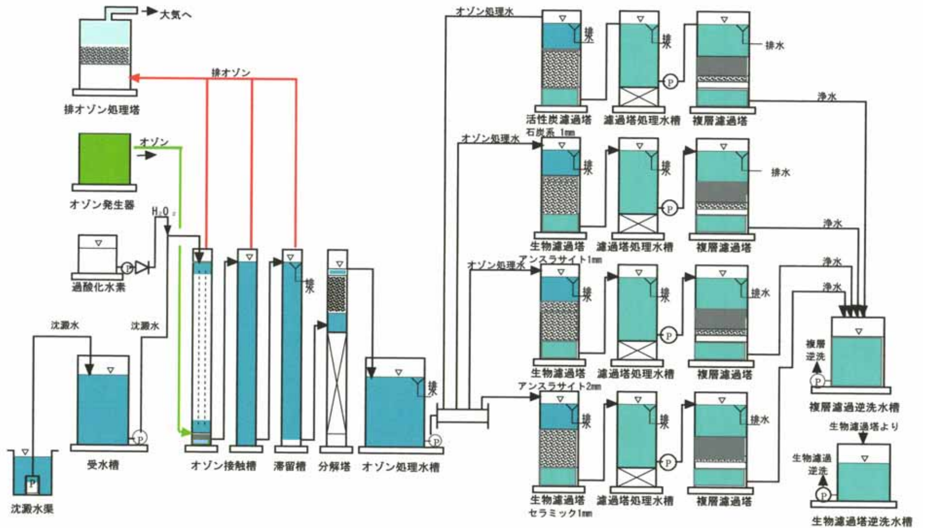
実証試験設備フローシート
